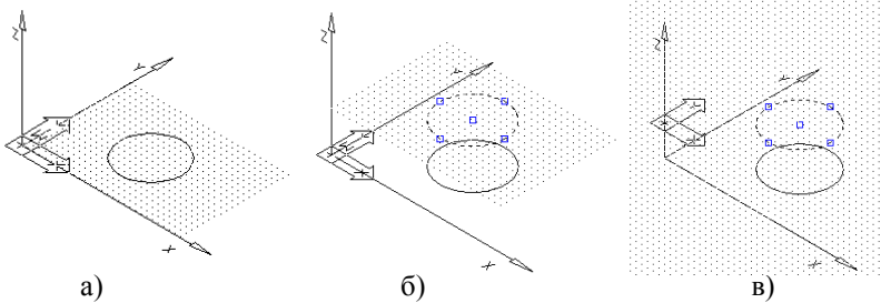
а) – построение окружности в мировой системе координат (МСК); б) - построение окружности в МСК, УРОВЕНЬ (ELEV) 100; в) - построение окружности в ПСК, созданной опцией Начало (Origin) или Перенеси (Move)
